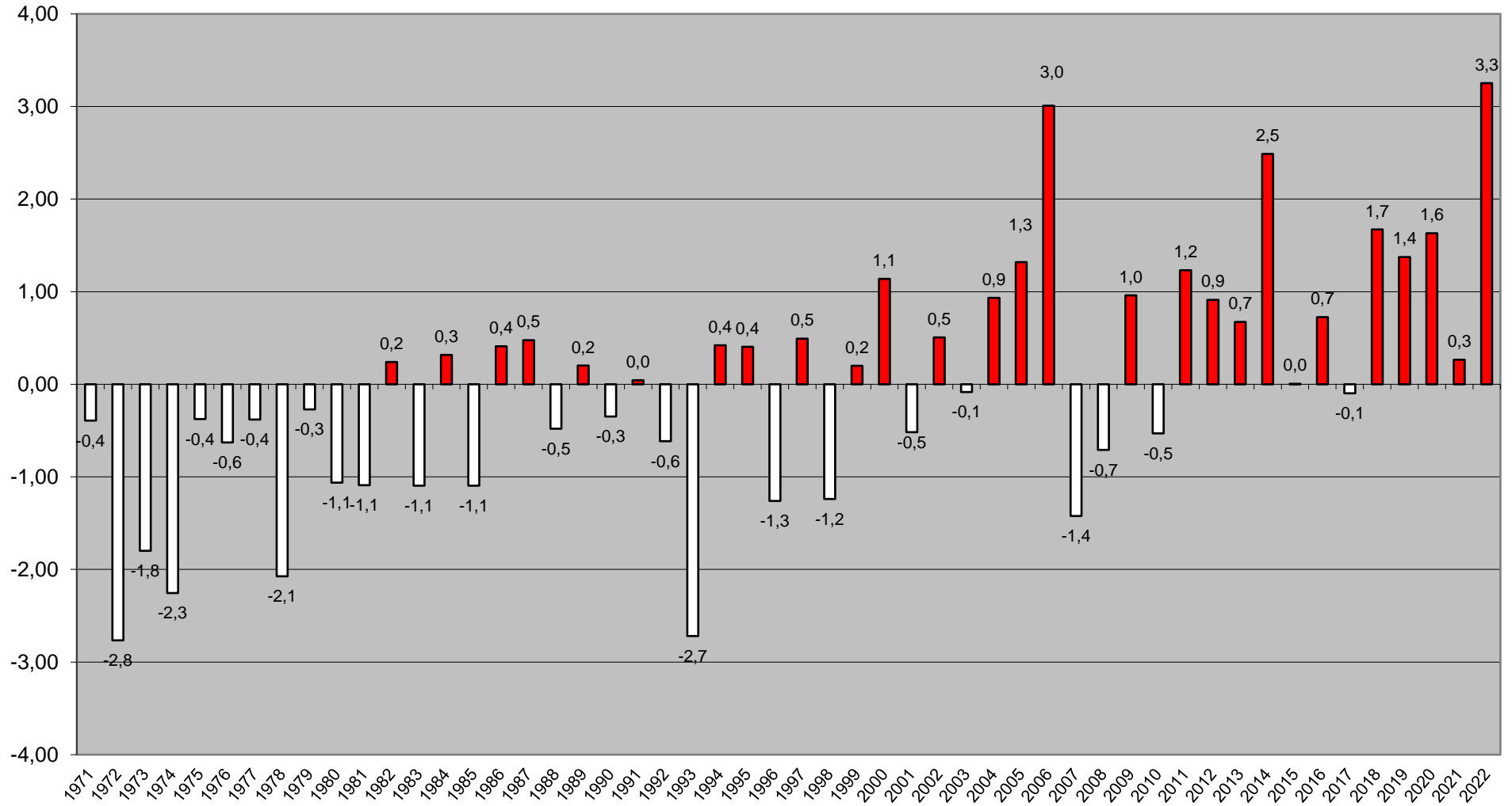
Ecart température moyenne automne ( septembre, octobre, novembre)
